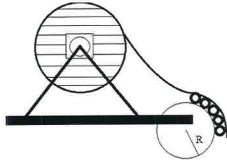
Rys. Ustawienie rolek podporowych z promieniem > od min. promienia gięcia kabla przy wejściu do kanału
